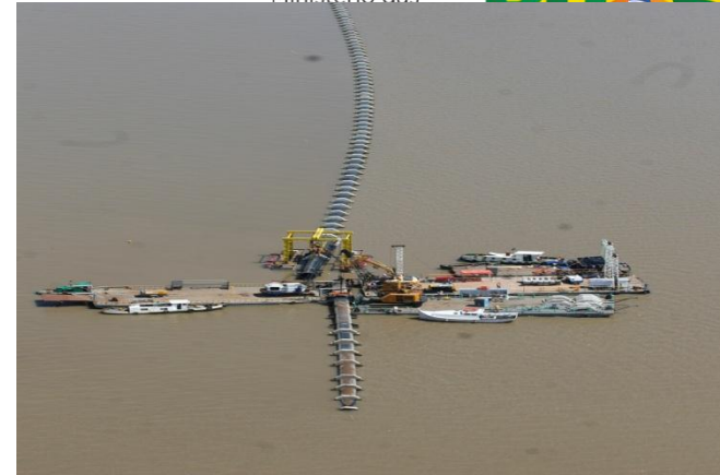
DESPOLUIÇÃO DOS VALES DOS RIOS DOS SINOS, GUAÍBA E GRAVATAÍ/RS Montagem do Emissário Subaquático – SES Ponta da Cadeia
